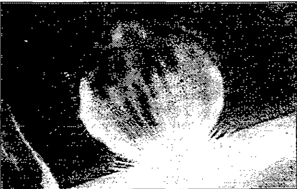
رسم يوضح خطورة سقوط النيازك على الكرة الأرضية
